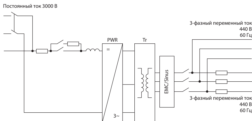
Рис. 25. Схема стандартного ПСН:
