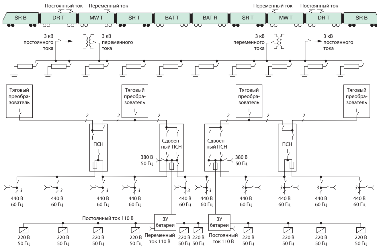
Рис. 23. Функциональная схема энергообеспечения собственных нужд
