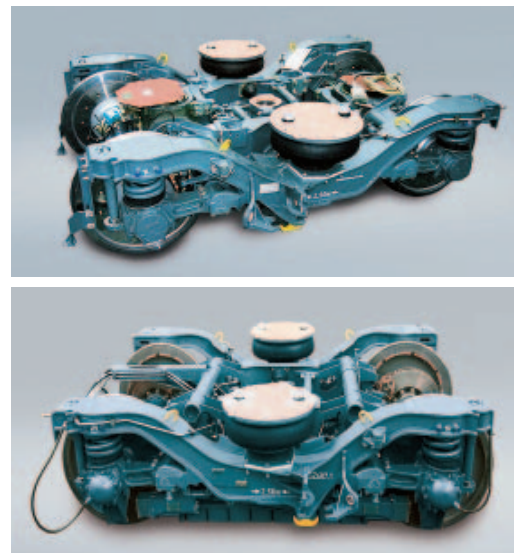
Рис. 8. Моторная (вверху) и немоторная тележки поезда Velaro RUS
