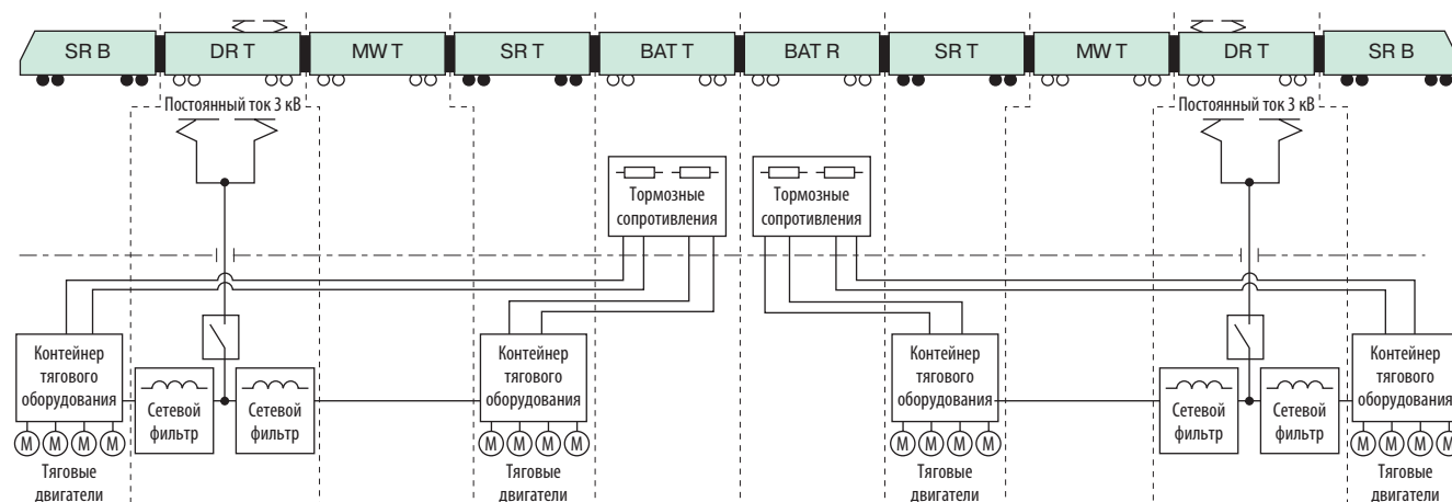
Рис. 12. Функциональная схема тягового оборудования односистемного поезда В1
